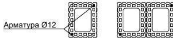
Рисунок 1. – Варианты армирования
